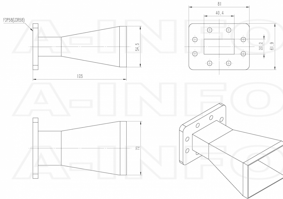
FDP58 Output (P/N: LB-159-10-A)
